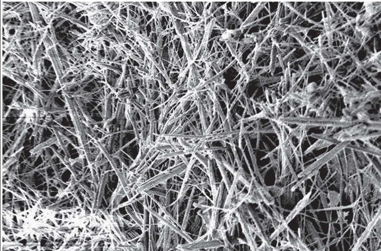
CALCESTRUZZO TRATTATO CON XYPEX
