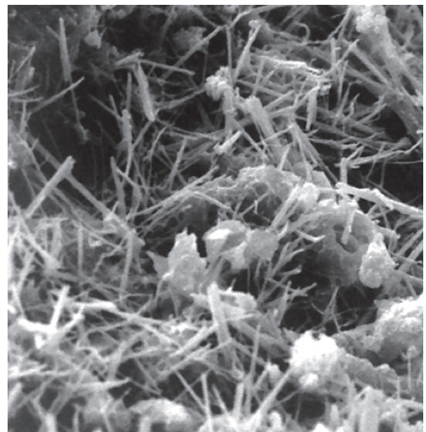
CALCESTRUZZO TRATTATO CON XYPEX
